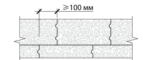
Рис. 4.4. Перевязка кладки
