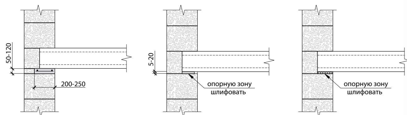
Рис. 4.13. Варианты перекрытий по стенам из блоков ЛСП
